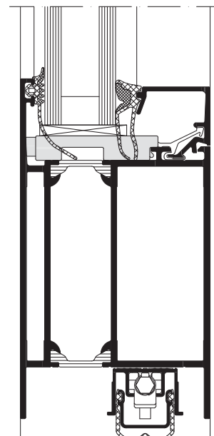
Schüco Tür-System ADS 75 HD.HI, Fußpunkt, Maßstab 1:2 Schüco door system ADS 75 HD.HI, Sill, Scale 1:2
